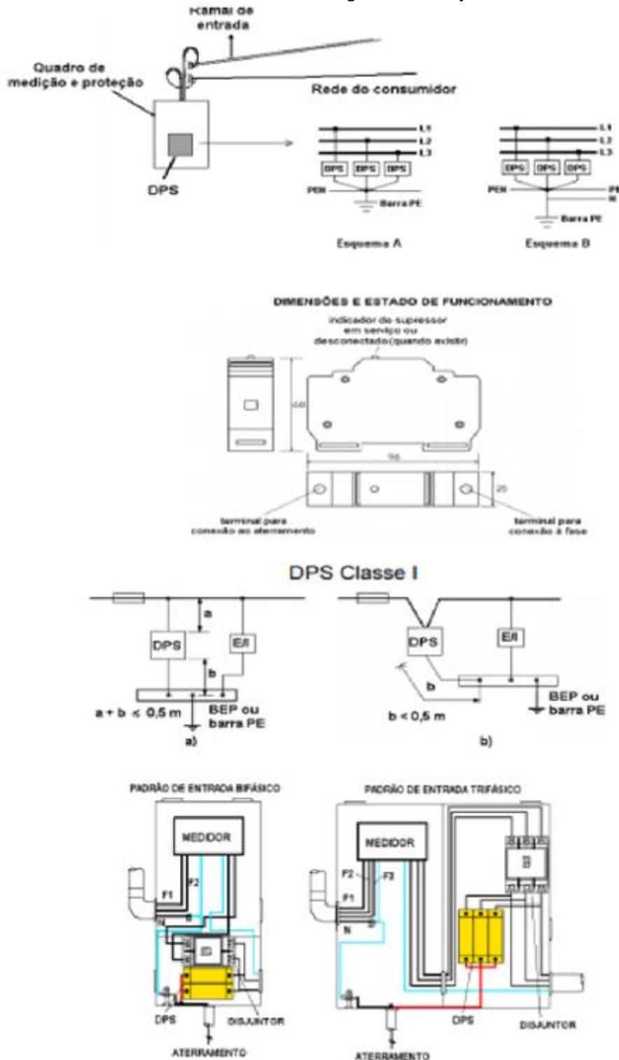
Figura 5 - Instalação do DPS
