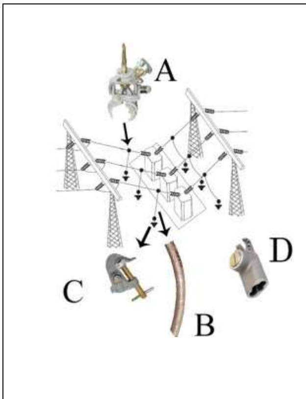
Figura 95 - Conjunto de aterramento temporário para subestação até 138kV
