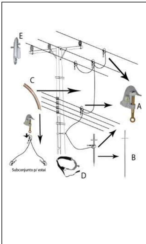
Figura 94 - Conjunto de aterramento temporário AT
