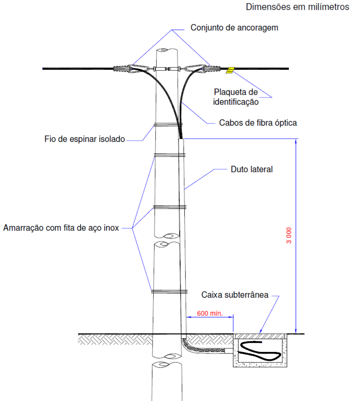
Figura 5- Caixa de emenda ou reserva técnica instalada em caixa subterrânea
